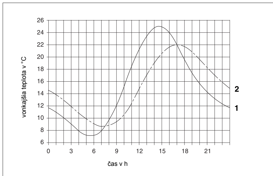
Obr. 15 Porovnanie aktuálnej a tlmenej vonkajšej teploty
