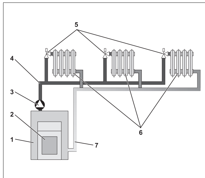
Obr. 1 Schéma vykurovania s núteným obehom (čerpádlom)
