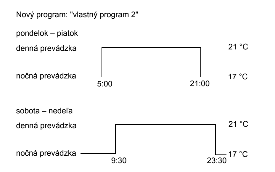
Obr. 20 Nový program vykurovania
