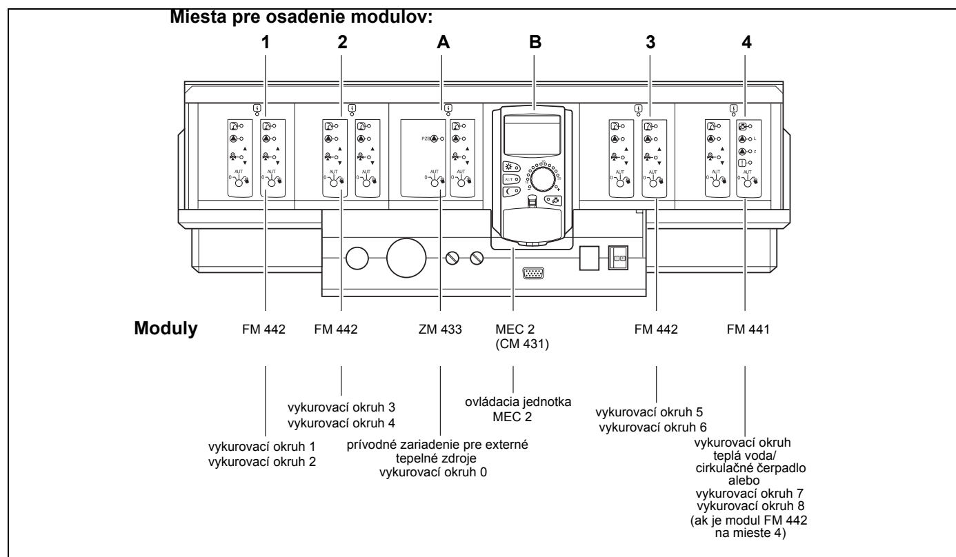
Obr. 5 Osadenie modulov (možná plná výbava)
