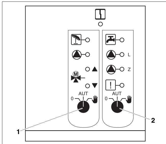
Obr. 24 Funkčný modul FM 441
