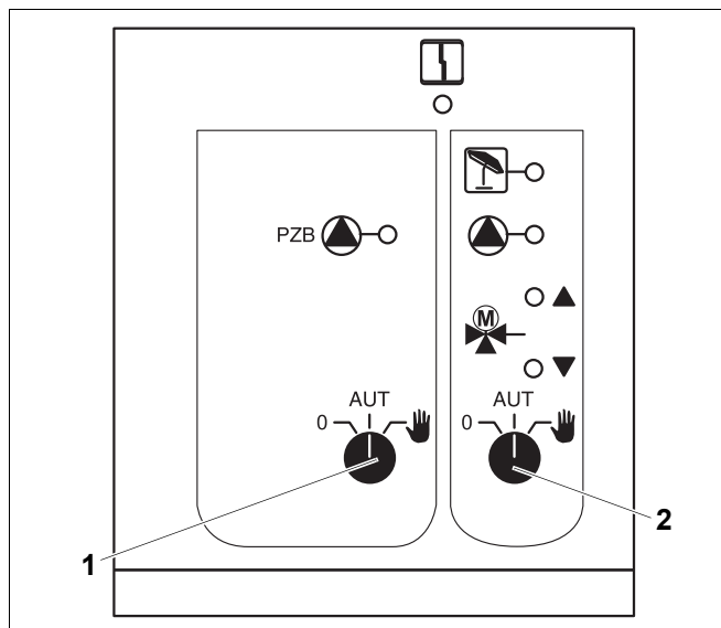
Obr. 22 Centrálny modul ZM 433
