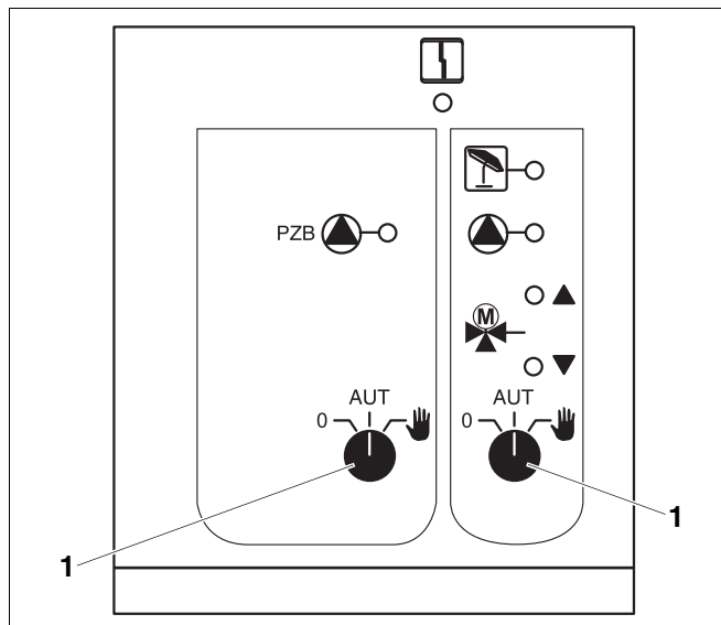
Obr. 8 Ručný spínač napr. na centrálnom module ZM 433
