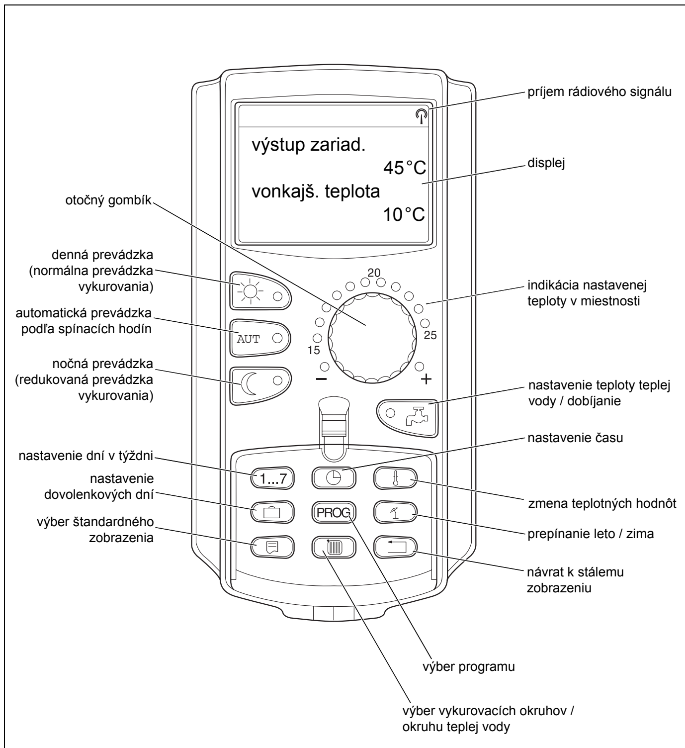
Obr. 6 Ovládacia jednotka MEC 2
