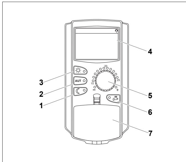
Obr. 7 Ovládacia jednotka MEC 2
