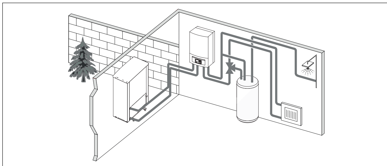
Obr. 3 Tepelné čerpadlo WPL AR, vnútrotná jednotka IDU E s elektrickou vložkou pre dohrev a externým zásobníkom teplej vody
