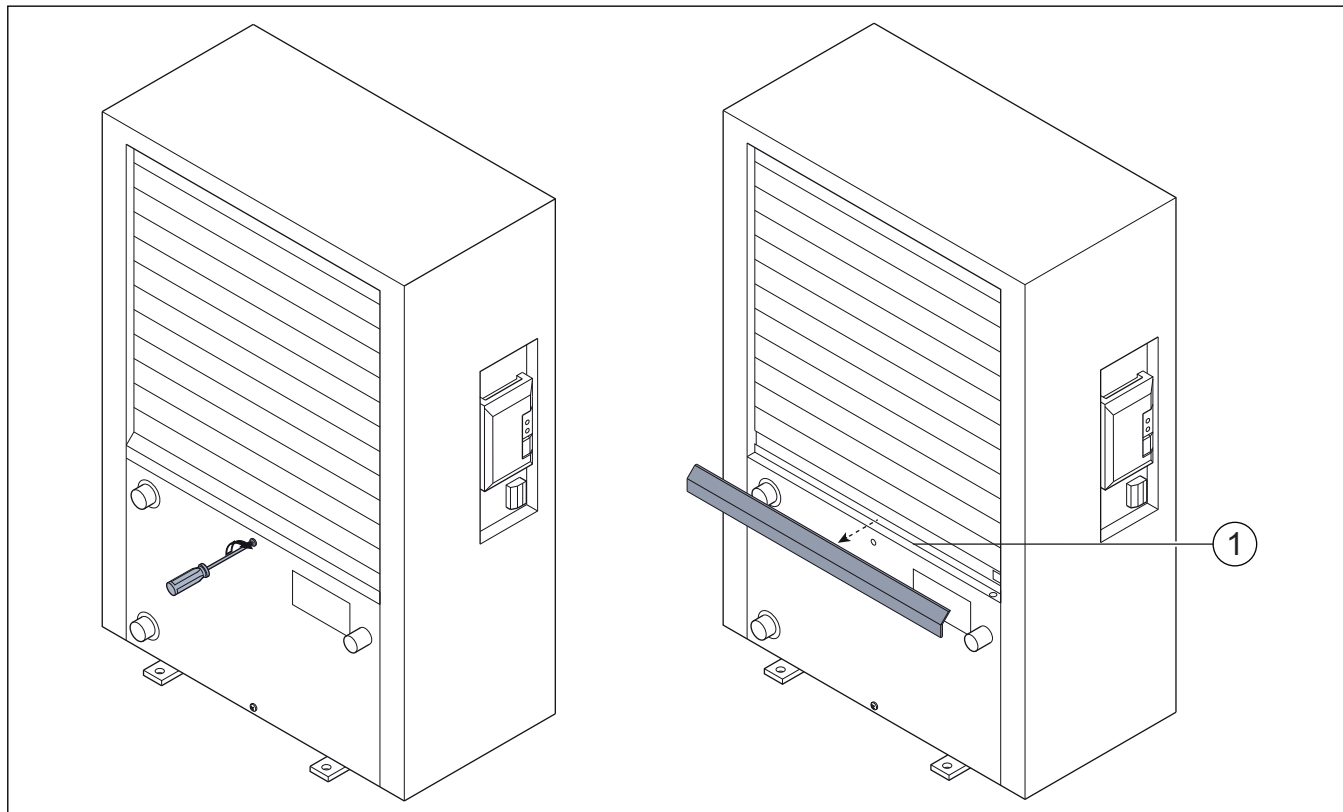
Obr. 8 Vaňa na kondenzát tepelného čerpadla
